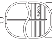
Одноотворный клапан (с сифонной трубкой) Жидкий хладагент должен заправляться, когда баллон стоит вертикально, как показано на рисунке.
